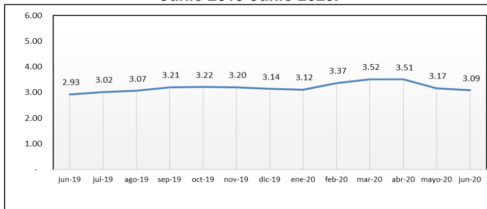
Gráfico N°12. Fondo Jubilaciones y Pensiones del Poder Judicial. Comparativo Riesgo Tasa de Interés-Duración Macaulay. Junio 2019-Junio 2020.
