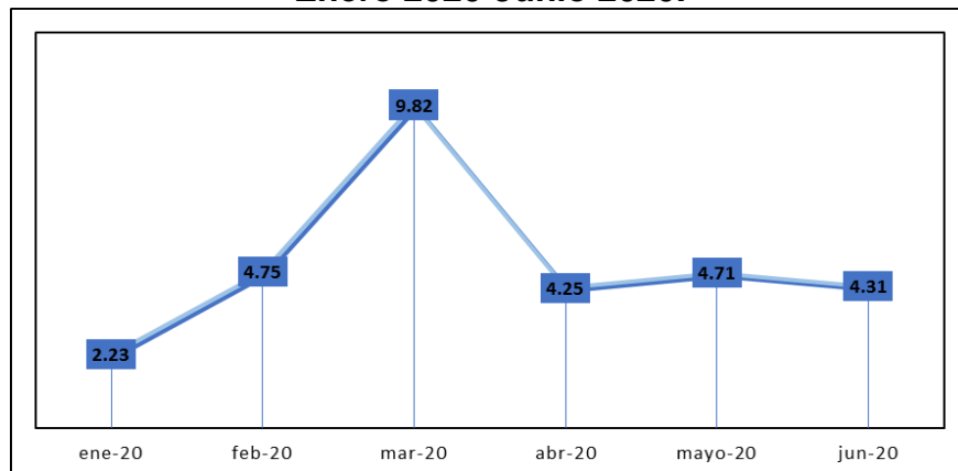
Gráfico N°22. Fondo Jubilaciones y Pensiones del Poder Judicial. Indicador de Cobertura de Liquidez. Enero 2020-Junio 2020.
