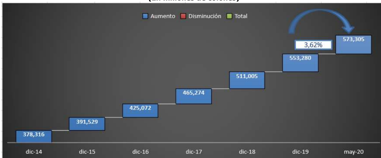
Gráfico 1 Valor Facial de Cartera Datos al 31 de mayo 2020 (En millones de colones)
